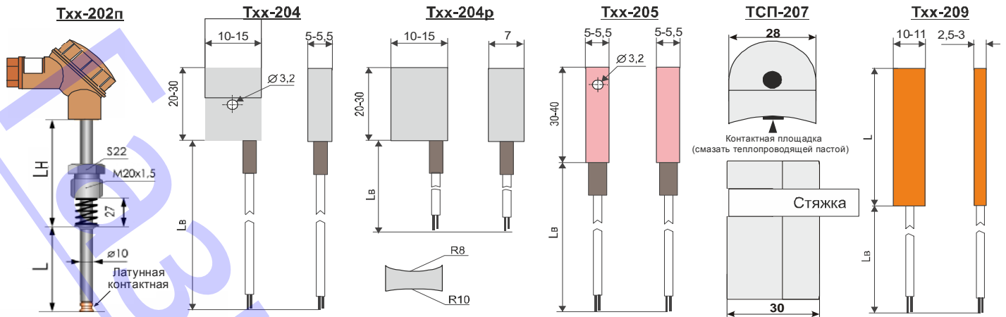
Рисунок 5 - Группа 2. Преобразователи поверхностные
