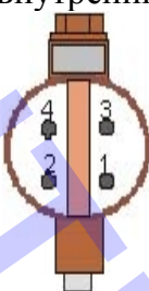
Рисунок 2 – Расположение клемм в контактной колодке
