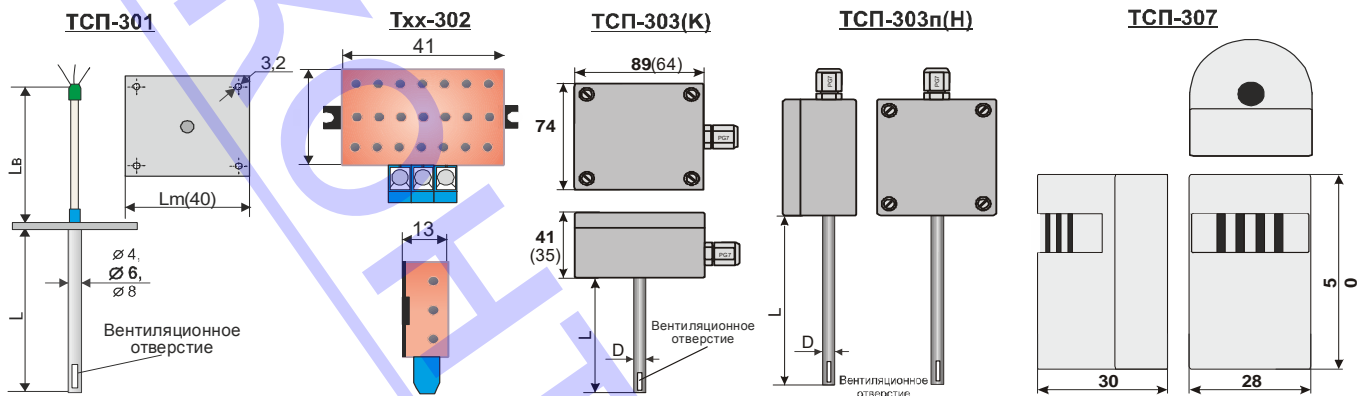
Рисунок 6 - Группа 3. Преобразователи воздушные
