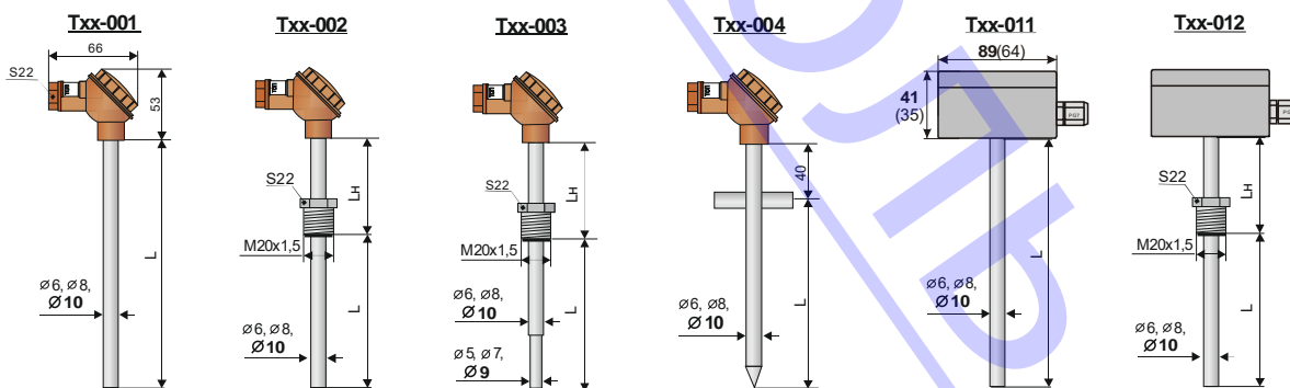
Рисунок 3 - Группа 0. Преобразователи погружаемые
