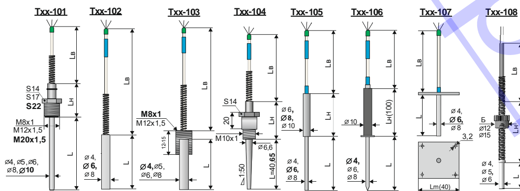
Рисунок 4 - Группа 1. Преобразователи погружаемые с кабельными выводами
